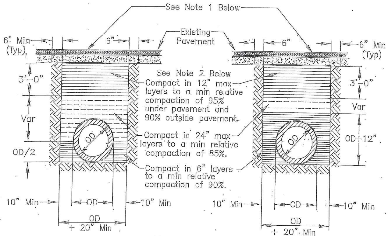
RIGID CONDUIT
